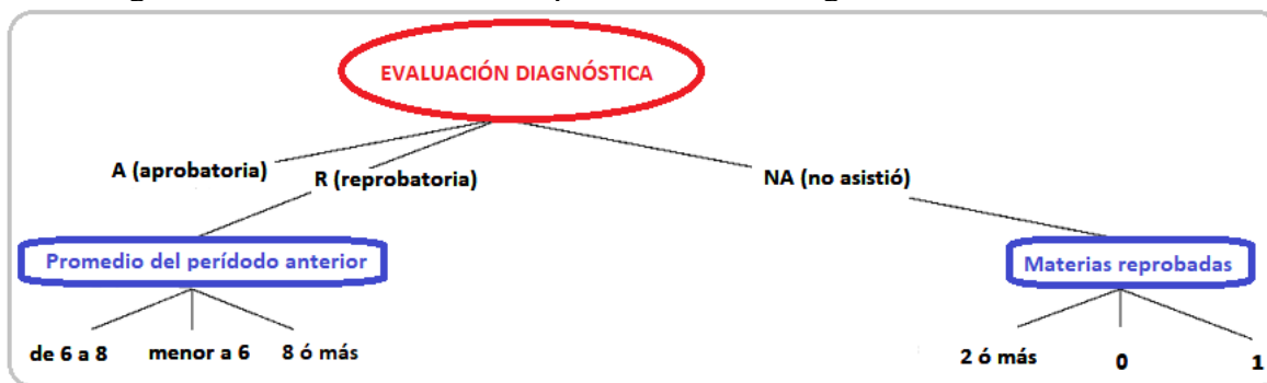
Figura 3. Estructura del modelo predictivo con el algoritmo árbol de decisión.
