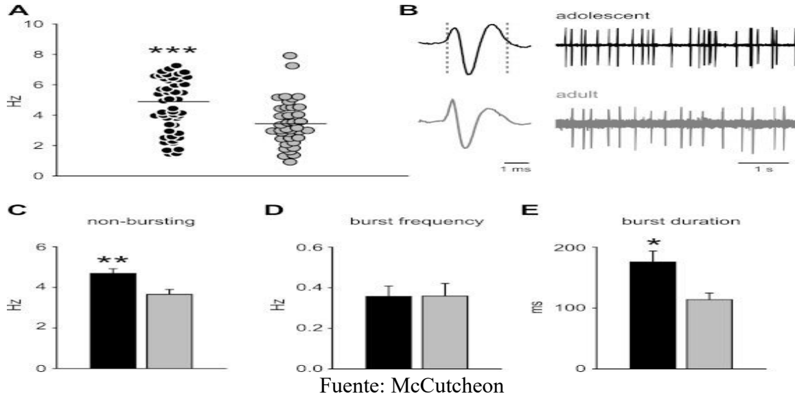
Figura 1. Las neuronas dopaminérgicas del área tegmental ventral (ATV) se disparan más rápido en ratas adolescentes que adultas.
